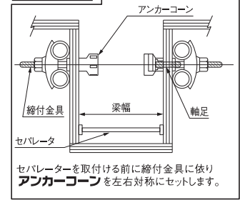
施工図(1)
