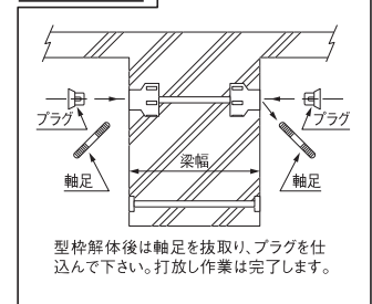
施工図(3)
