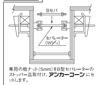
施工図(2)
